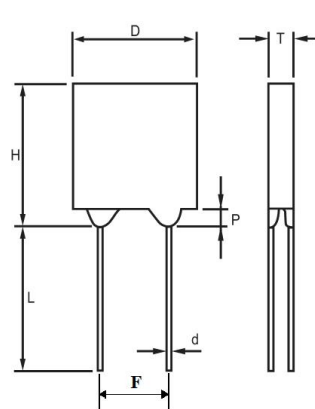
(图 3: 方形产品简图)
